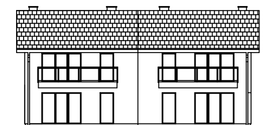
ELEWACJA OGRODOWA
