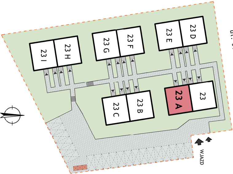
SCHEMAT ZAGOSPODAROWANIA TERENU
