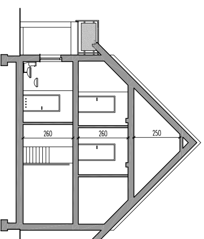
PRZEKRÓJ
