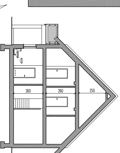
PRZEKRÓJ
